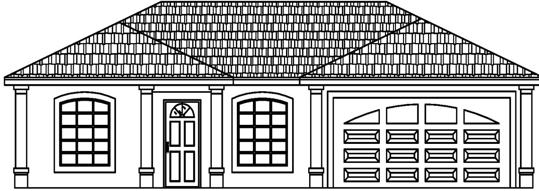
ELEVATION A
