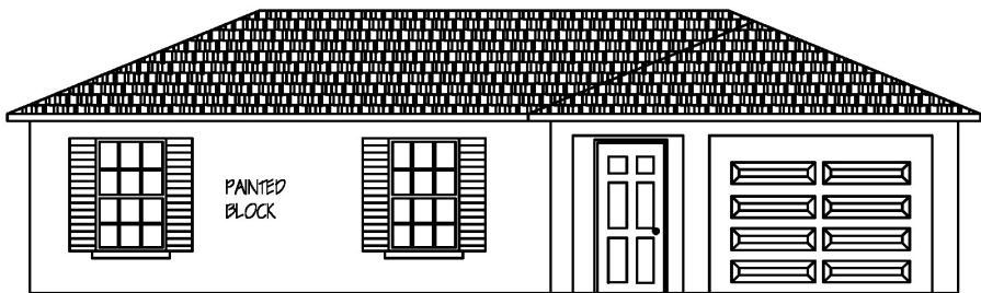
ELEVATION A
