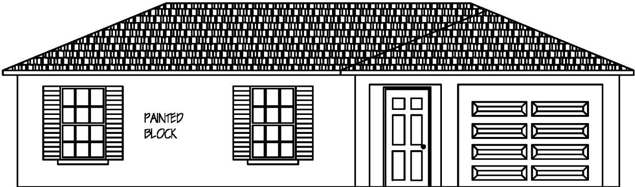
ELEVATION A
